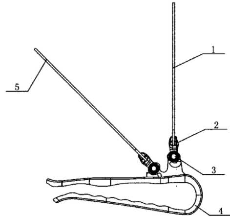
圖 11. 多功能遮陽板設計圖
