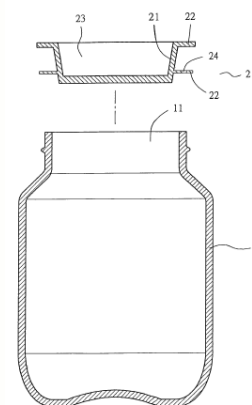
圖 10. M480818 瓶蓋在未置入容器開口的截面示意圖
