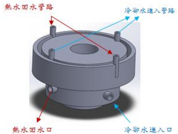
圖 7. 軸向旋轉式冷卻水循環系統
