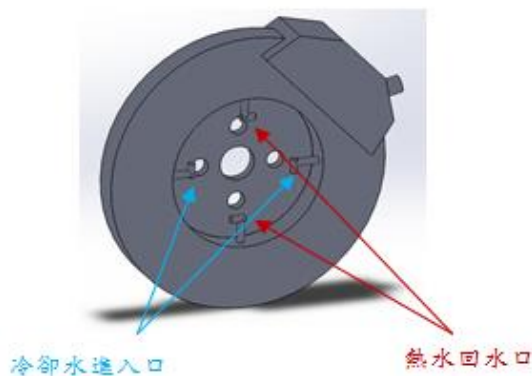
圖 6. 76 內含冷卻水道之碟盤
