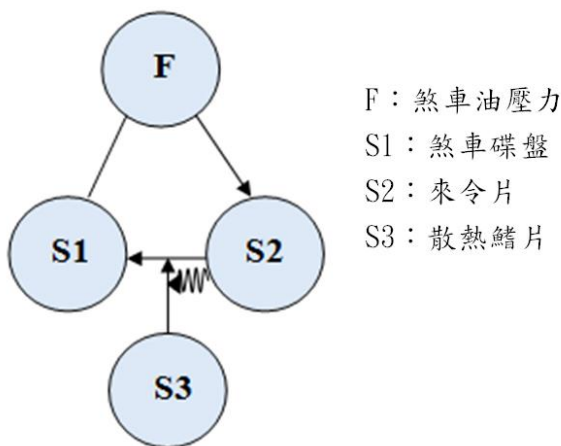
圖 5.76 標準解之解決模型
