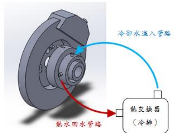
圖 8. 分離水冷式碟式煞車系統
