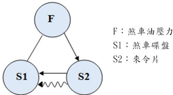
圖 4.物質一場分析模型
