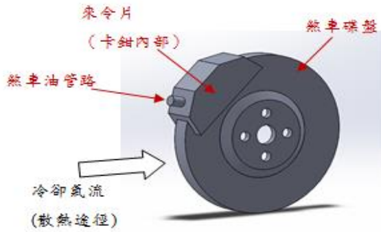
圖 1. 碟式煞車之散熱系統的簡易示意圖
