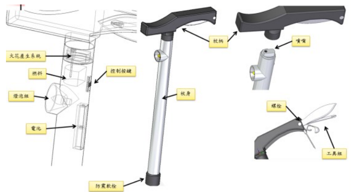
圖 18. 整合後設計藍圖
