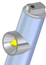
圖 16. 登山杖固定噴嘴、燈泡組後圖
