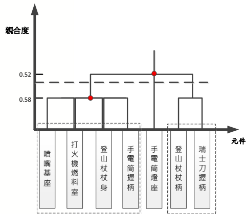
圖 14. 分群枝狀圖(0.52至0.58)
